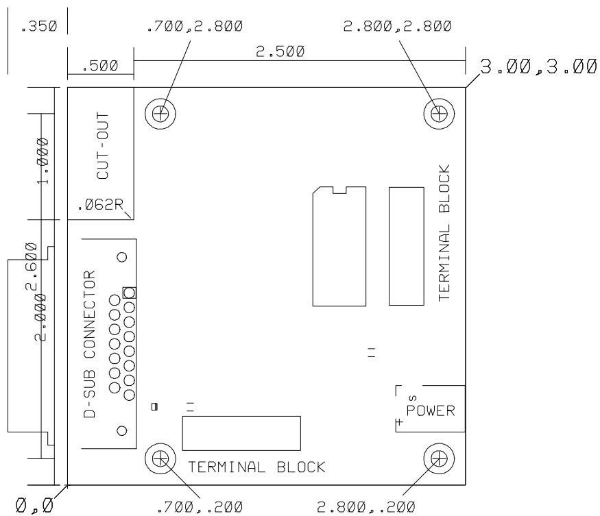
ROKU_HD_4X4 LAYER 14, TEST FIXTURE BLOCK
